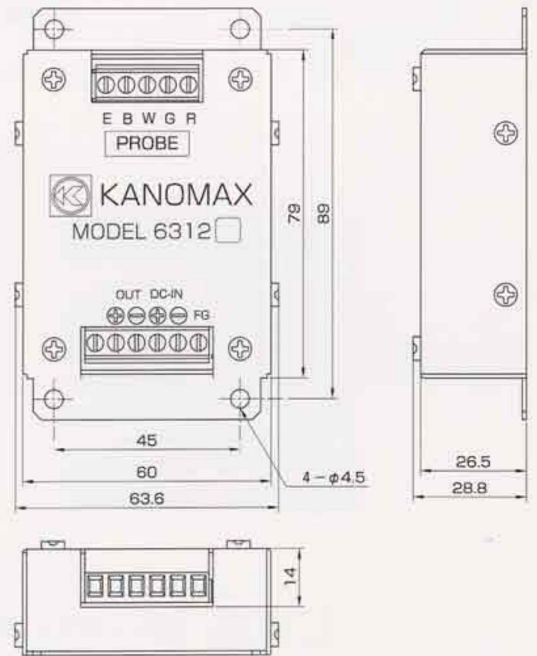
■収納BOX外観寸法
