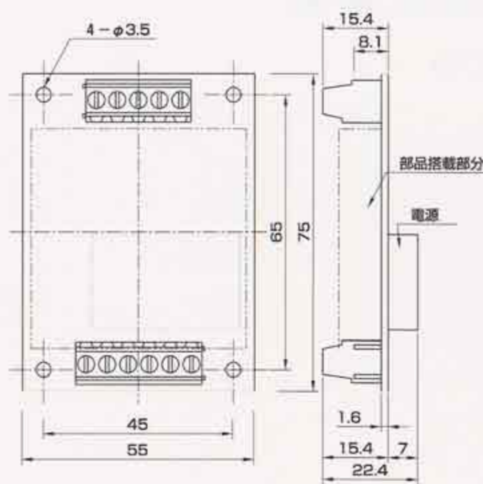
■本体外観寸法
